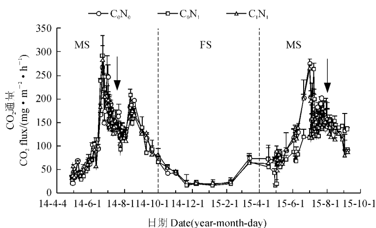
图 2 不同处理旱作春玉米农田 CO 2 通量动态变化
