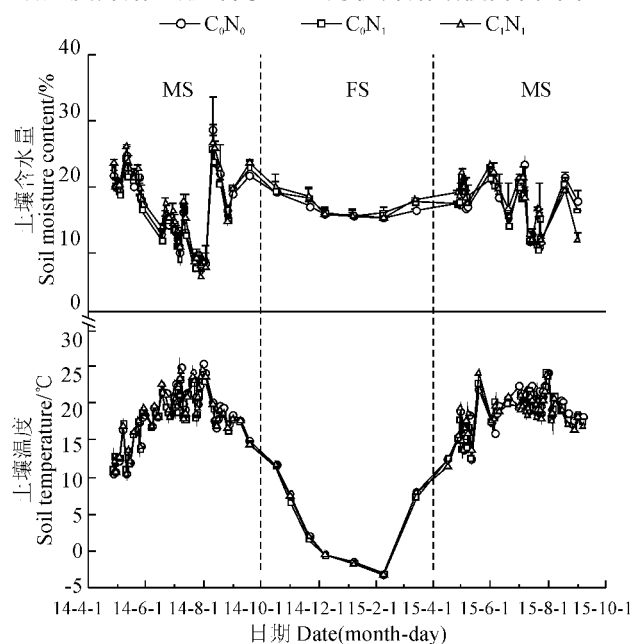
图4 旱作春玉米农田土壤水分及温度的动态变化
