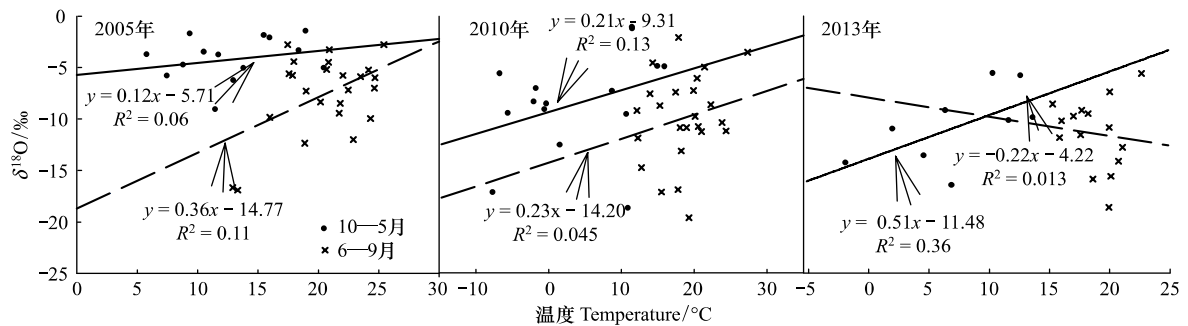
图4 降雨 \delta^{18}\text{O} 与温度的关系
