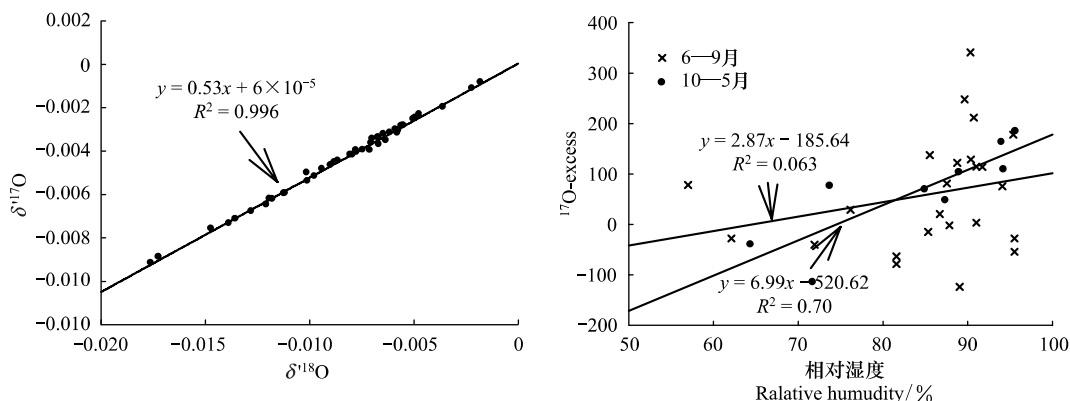
图 7 氧同位素降水方程线与 ^{17}\text{O} 盈余和相对湿度的关系
