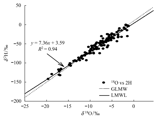
图5 大气降水 \delta\text{D} 和 \delta^{18}\text{O} 的关系
