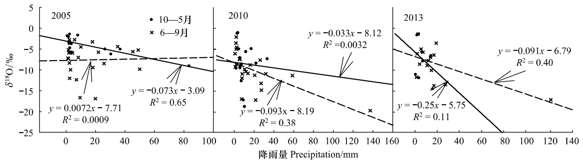
图3 降水量与 \delta^{18}\text{O} 的关系
